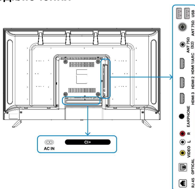
Рисунок 1 – Терминалы задней панели телевизора
