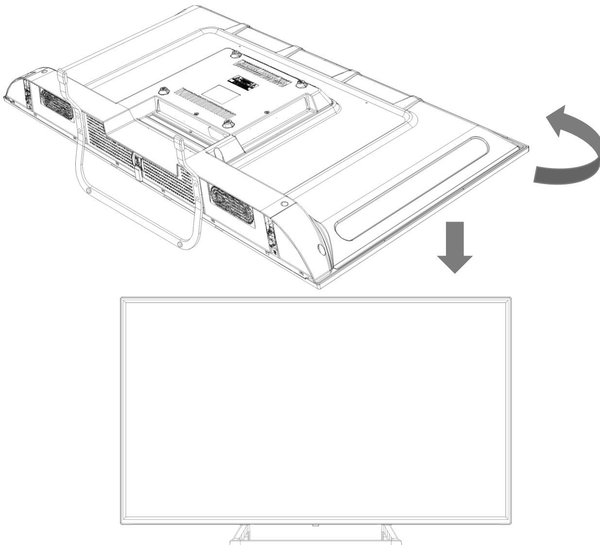
Рисунок 6 – Установка телевизора на центральной опоре
