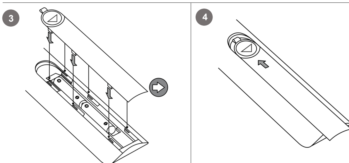
Рисунок 45 – Установка элементов питания в пульт ДУ
