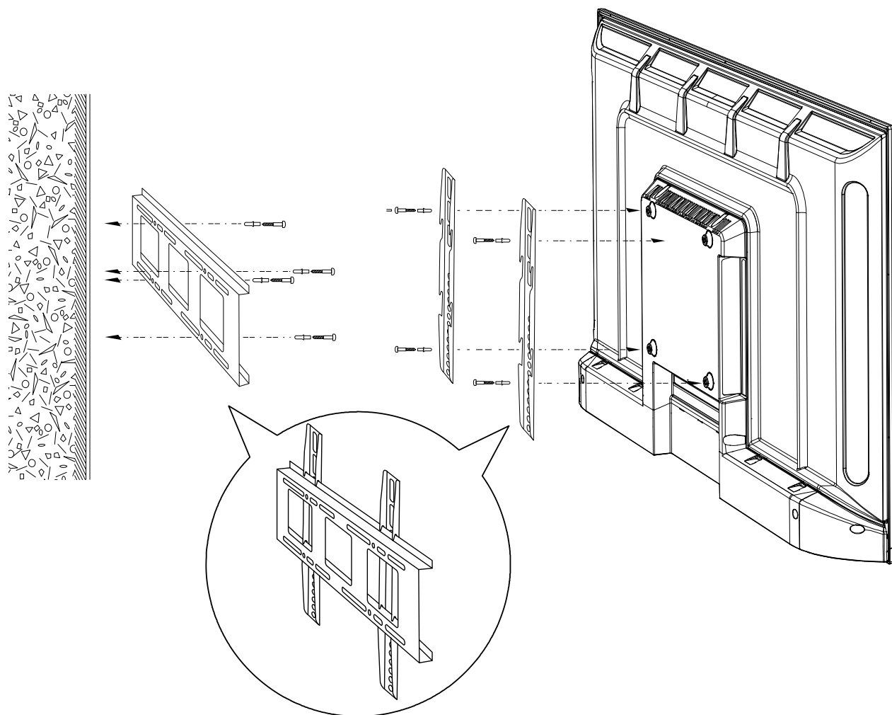
Рисунок 7 – Настенный монтаж телевизора
