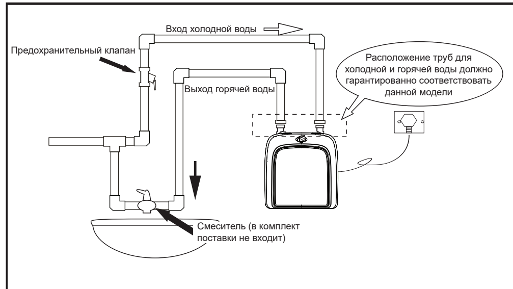
Монтажная схема для моделей, как серии Q2/Q2C/RQ2, у которых горячая вода поступает наверх.
